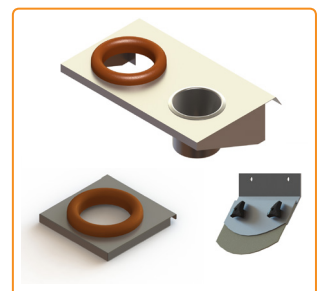
Intégration réceptacle à liquide Raclette à déchets fixation sur table Bloc de tri avec TVO en saillie
