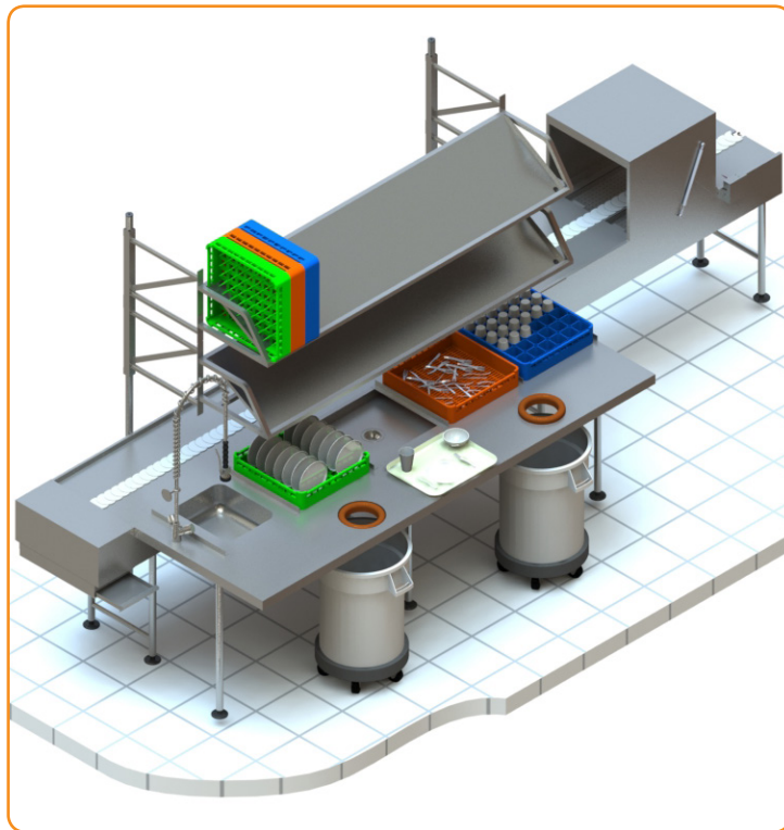
Goulotte à couvert pour table de triage Code : G22
