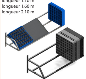
Etagère de horizontale Etagère entrée machine inclinable
