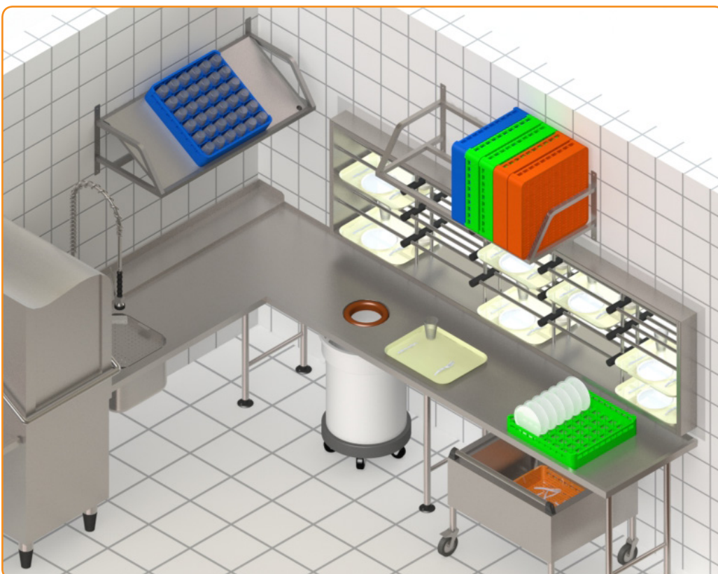
Intégration réceptacle à liquide Raclette à déchets fixation sur table Bloc de tri avec TVO en saillie
