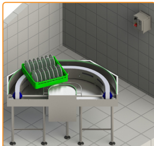
Virage 180° motorisés
