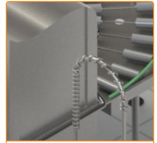
4 ensemble de 2 mini-rouleaux inox pour virage après tunnel de séchage
