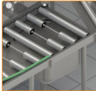
Élément de 0.5 m avec bac incorporé de 400x400x300 panier filtre et support douche
